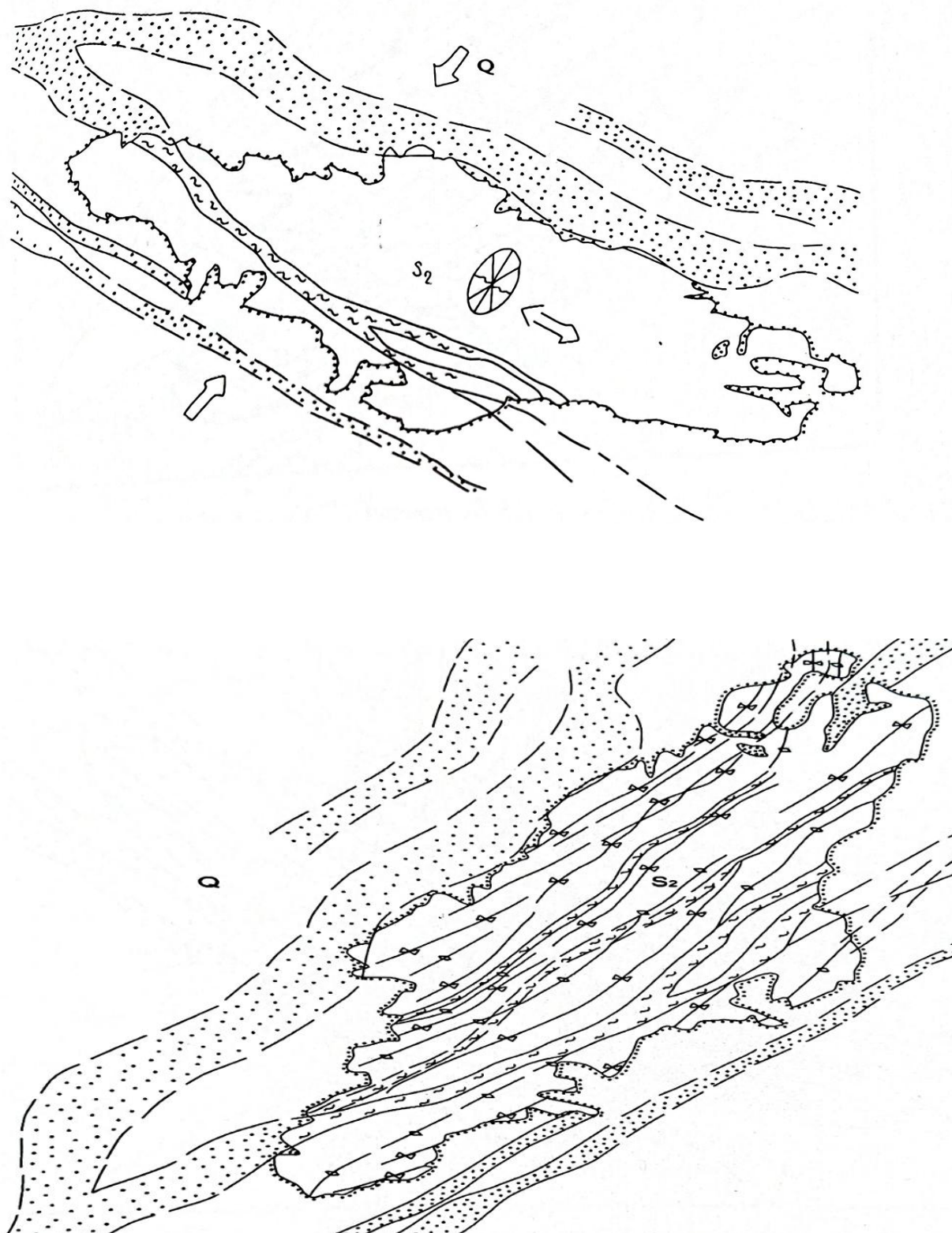
Рис.1. Схема развития структуры рудного поля Марджанбулак (По материалам Д.В.Шныреву)
