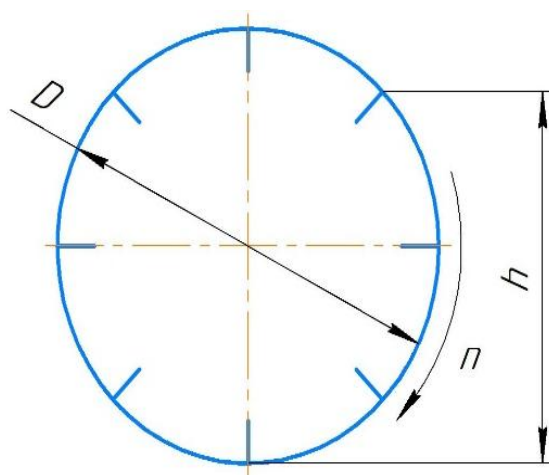
Рисунок 3. Расчётная схема барабанной сушилки
