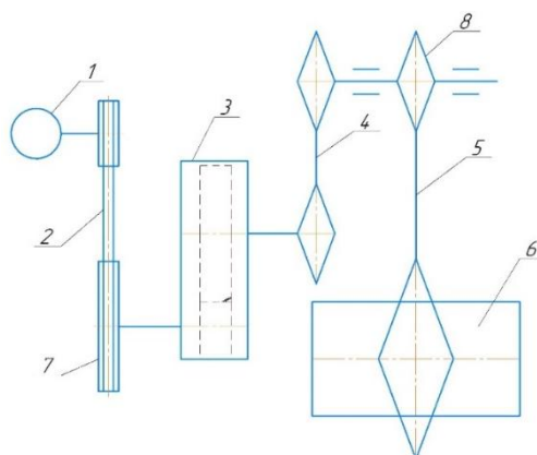
Рисунок 1. Кинематическая схема привода цепной передачи предложенный к малогабаритный сушильный барабан.
