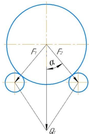
Рисунок 2. Схема действия сил на катки
